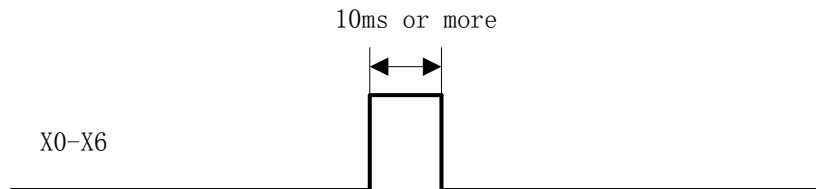
X0-X6 时序图
